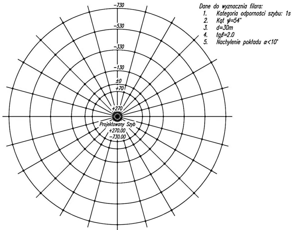
Rys. 16.2 Rzut poziomy projektowanych warstw filara szybu
