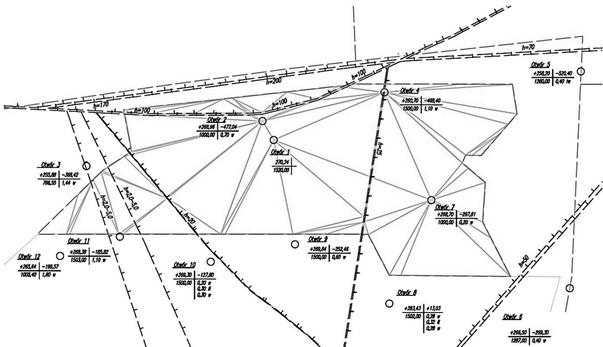
Rys. 16.6 Powierzchnia TIN spągu pokładu uwzględniająca uskoki
