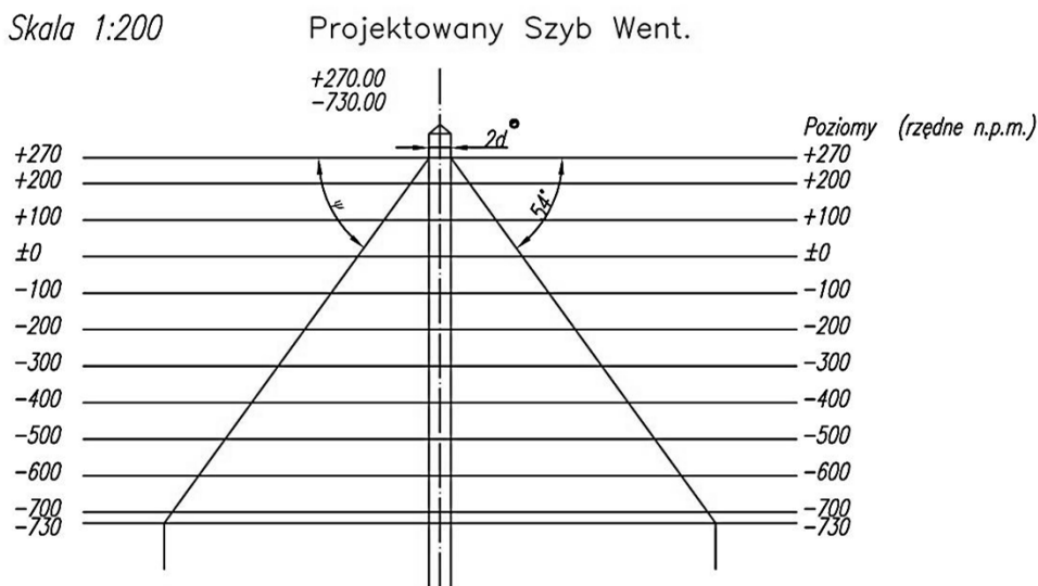
Rys. 16.1 Przekrój pionowy projektowanego filara szybu
