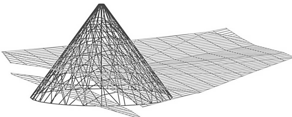
Rys. 16.8 Wizualizacja numeryczna bryły projektowanego filara szybu wraz z numerycznym modelem spągu pokładu w strefie uskokowej
