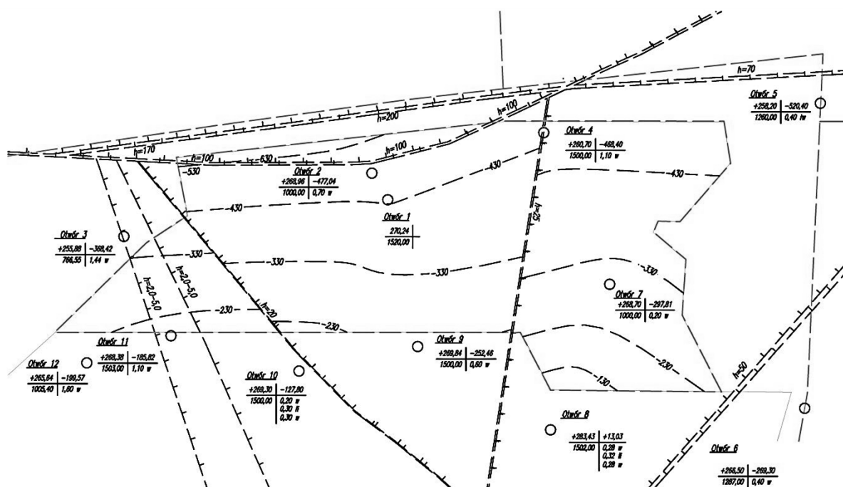
Rys. 16.5 Dokumentacja geologiczna wykorzystana do utworzenia powierzchni spągu pokładu
