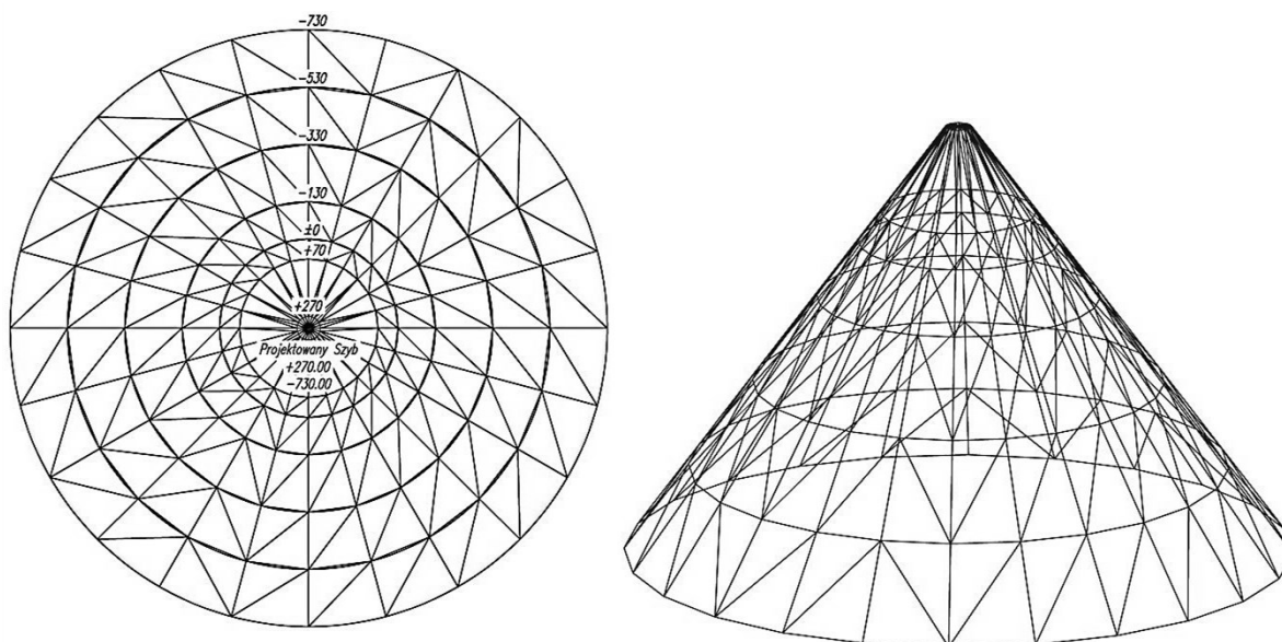
Rys. 16.4 Powierzchnia TIN projektowanego filara, rzut z góry i boku
