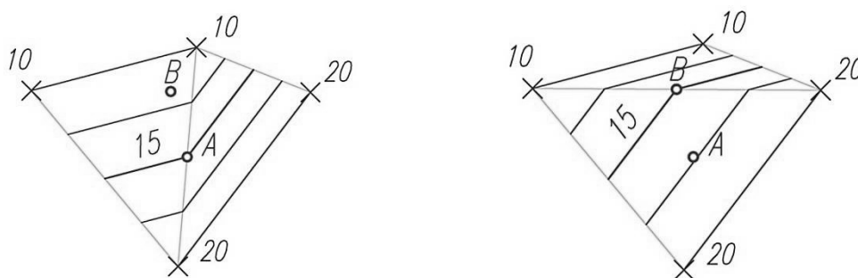
Rys. 16.3 Wpływ budowy trójkątów na interpolację warstw
