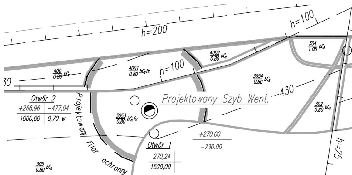
Rys. 16.9 Wyznaczony filar ochronny dla szybu
