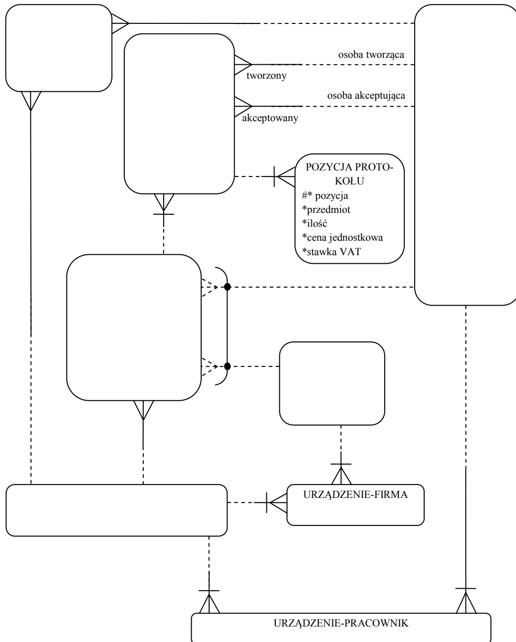
Rys. 8.1 Diagram ERD dla omawianego problemu
