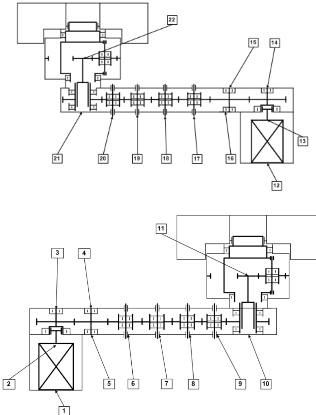
Rys. 4.8 Schematy kinematyczne ramion kombajnu ściany Eickhoff SI-300, z zaznaczonymi punktami pomiarowymi
