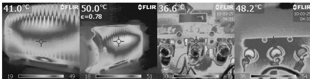
Rys. 4.3 Przykładowe termogramy przedstawiające rozkład temperatury na powierzchni obudowy, oraz zabezpieczenia przeciążeniowego transformatora It 3Sb
